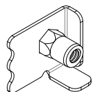
k) (1) Attache de garde-boue Côté passager Pièce n° 769313
